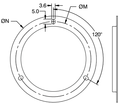
BF - BACK FLANGE
